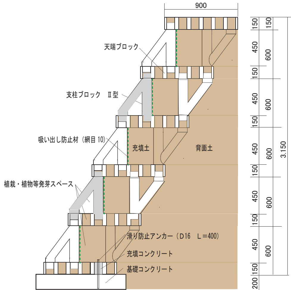
断面図（A～A'）
