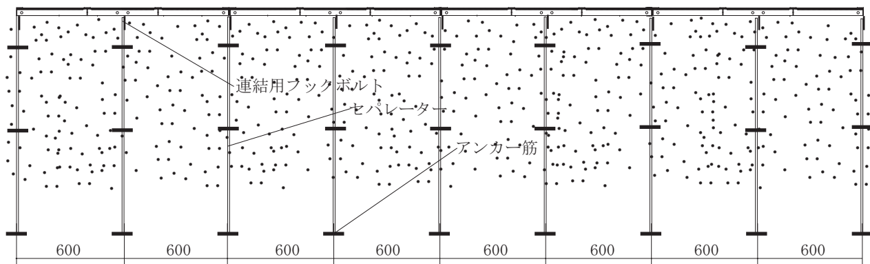
B~B' 断面図
