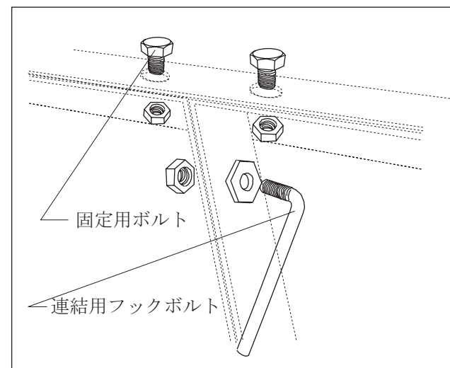
連結用フックボルト 組立詳細図
