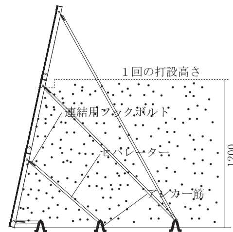
A~A' 断面図
