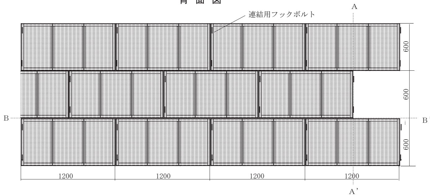
背面図
