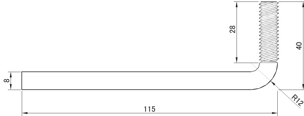
据付部品
