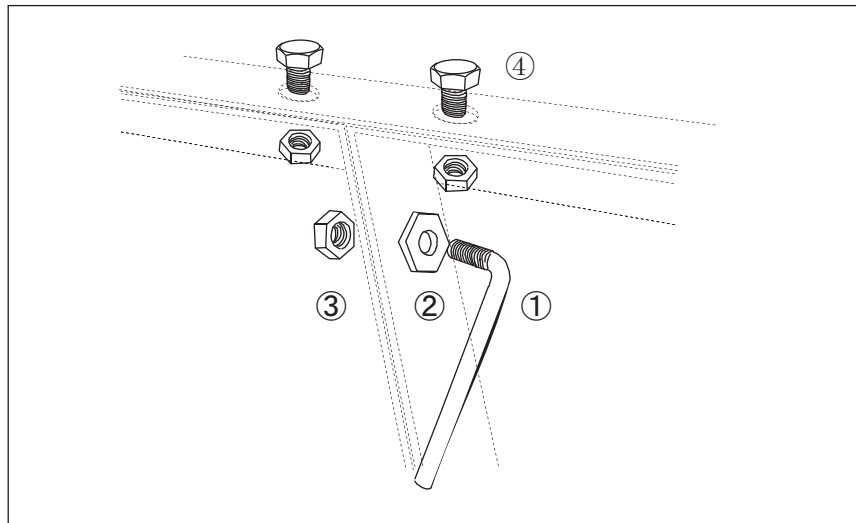
据付部品
