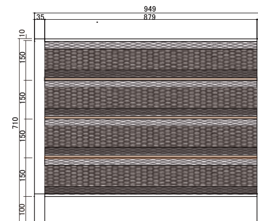
90° 4段プランター
